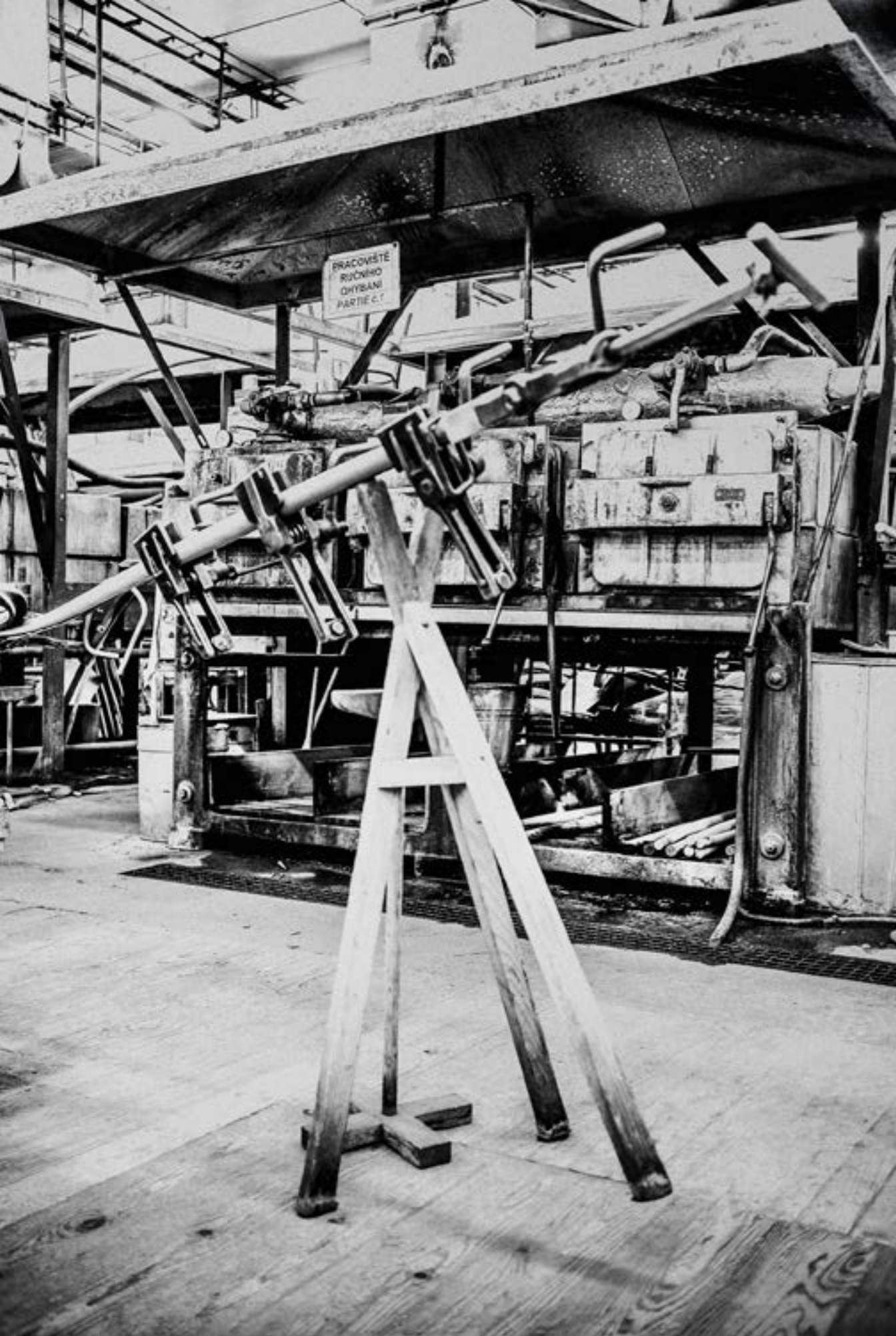
cz Trojnožka, která slouží pro odložení částí ohybu židle č. 14 a 18 en Tripod used for setting aside parts of backrests for chairs No. 14 and 18 de Dreibeinstuhl für das Ablegen eines Biegeteils für den Stuhl Nr. 14 und 18 pl Statyw podtrzymujący jeden z giętych elementów krzesła nr 14 i 18
